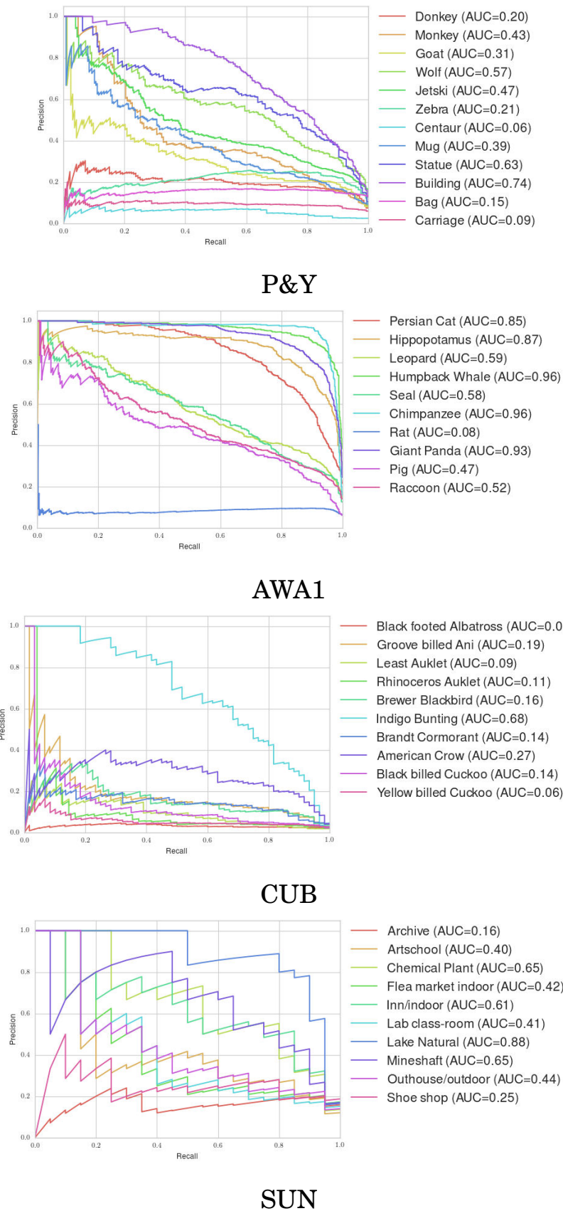
FIGURE 1.17 – Courbes de précision rappel.
