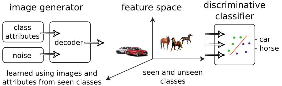
FIGURE 2.5 – La génération de caractéristique image \hat{\mathbf{x}} est conditionnée par : la représentation sémantique \mathbf{a} et un échantillon aléatoire d’une distribution multivariée \mathbf{z} . Après génération, un modèle de classification \hat{y} = f_D(\mathbf{x}; \hat{\mathcal{D}}_u, \mathcal{D}_s) peut être optimisé avec supervision pour les classes vues et non vues.
