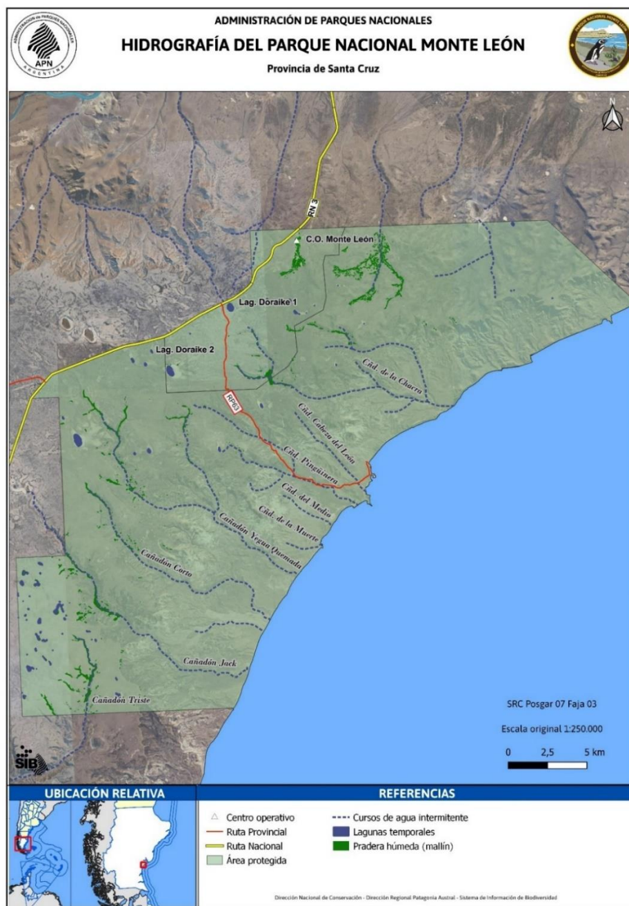
Figura 4. Hidrografía del PNML
