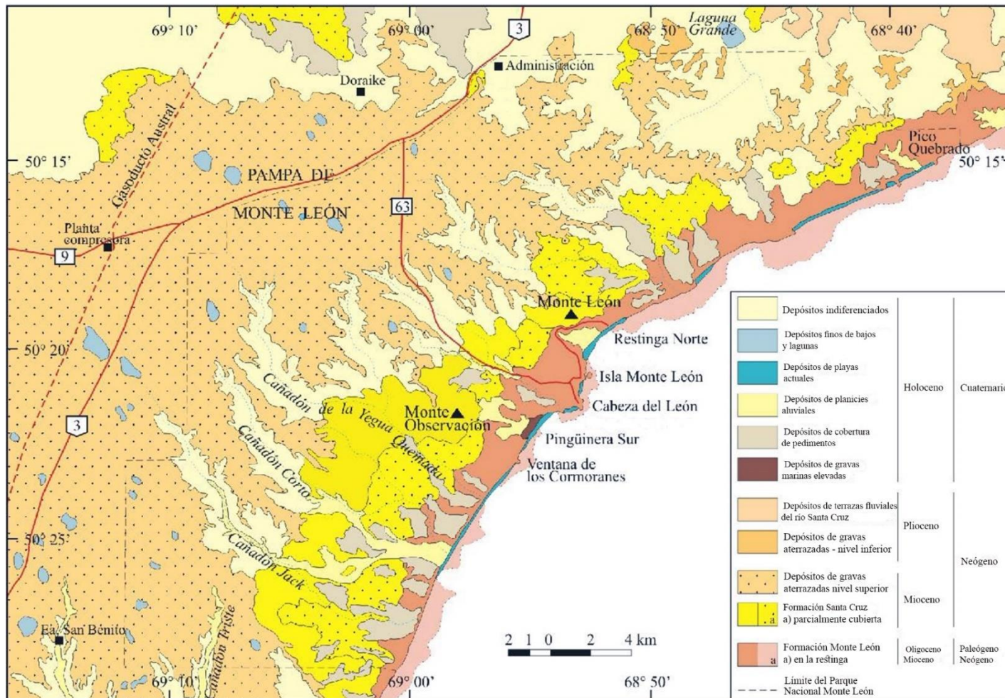
Figura 7. Mapa geológico del PNML. (Tomado y modificado de Sacomani et al. 2012: Figura 2).
