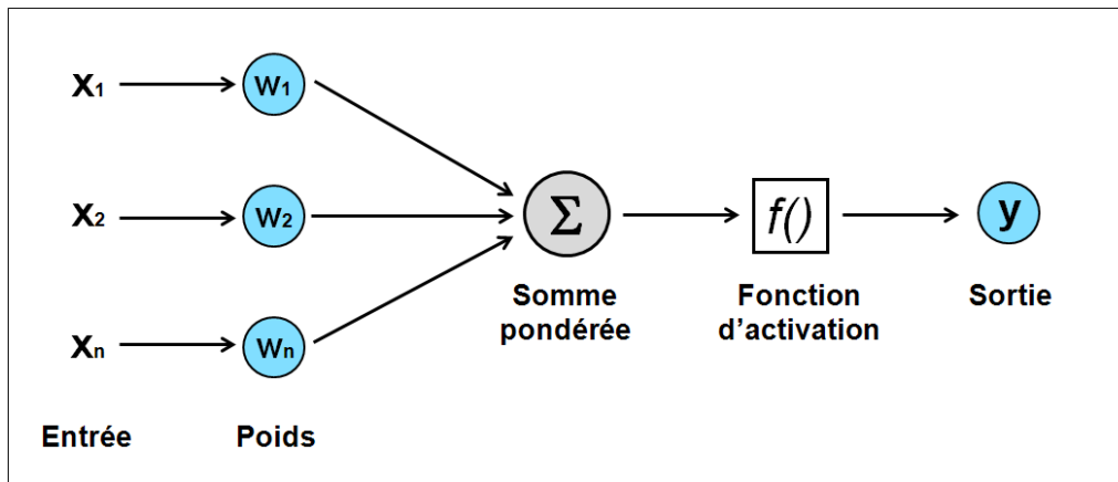
FIGURE 5.7 – Principe de fonctionnement d'un neurone formel
