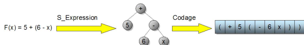
Figure 117 : Codage chromosomique basé sur les S_Expressions
