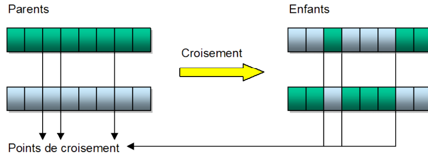
Figure 119 : Croisement uniforme de deux chromosomes
