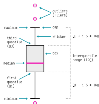
Figura 22: Anatomía de un diagrama de caja 14
