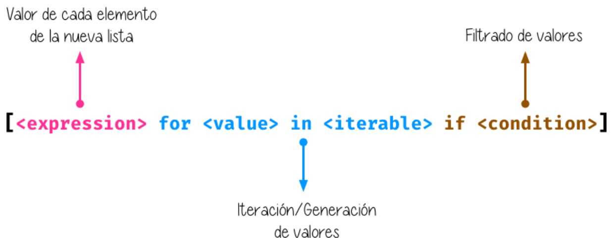
Figura 2: Estructura de una lista por comprensión
