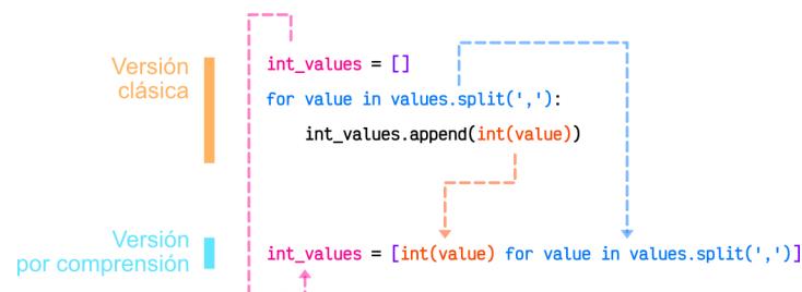
Figura 3: Transformación de estructura clásica en lista por comprensión
