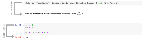
Figura 1: Ejecución de celdas en Jupyter Notebook
