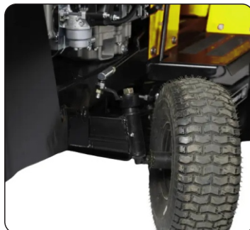
Ruedas y ejes de dirección sobre bujes de nylon PA-30GF, con alemite 1/4 para su correcta lubricación con grasa.
